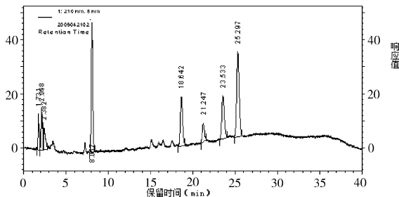
图3 供试品的HPLC色谱图 (C 8 )
