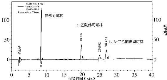
图2 对照品的HPLC色谱图 (C 8 )
