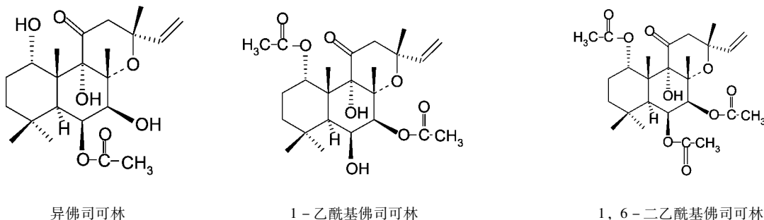
图 1 异佛司可林, 1-乙酰基佛司可林, 1,6-二乙酰基佛司可林的化学结构
